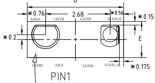
正视图
