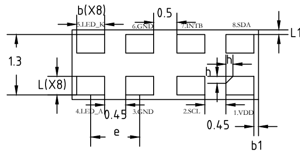
背视图
