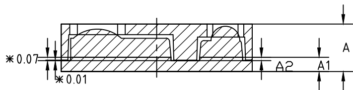
侧视图
